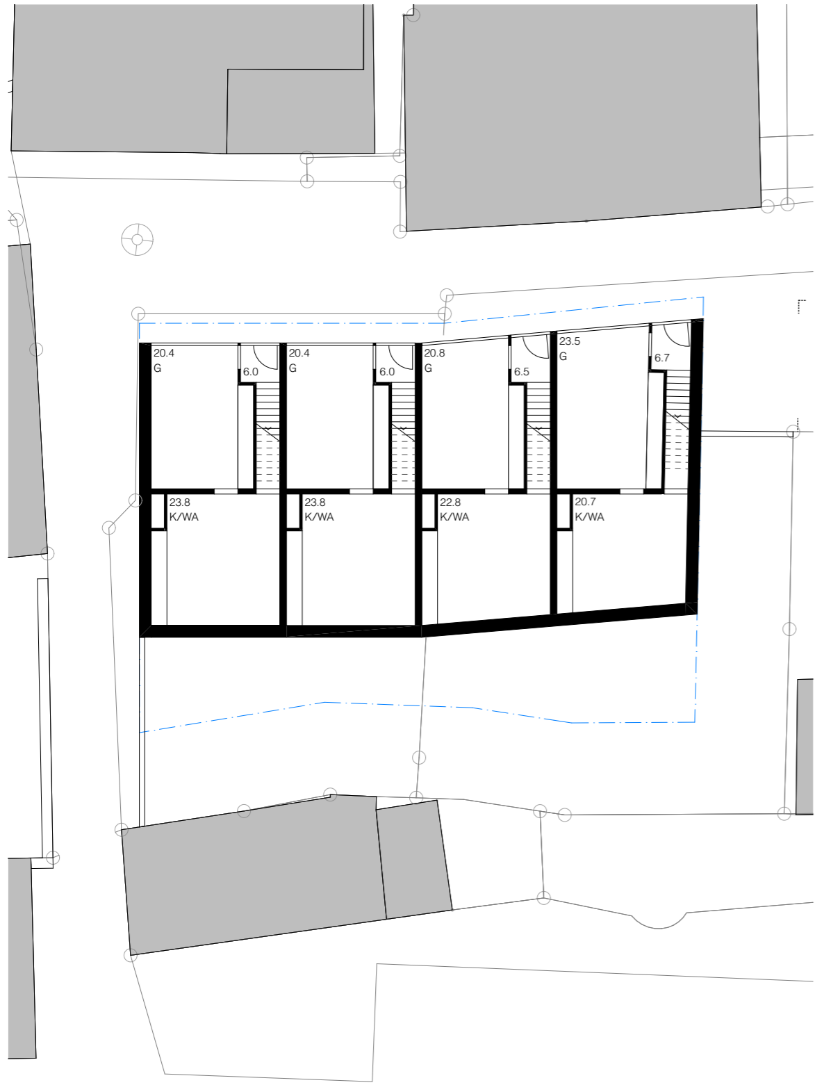
Erdgeschoss
